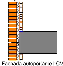
Fachada autoportante LCV
