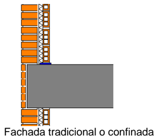
Fachada tradicional o confinada
